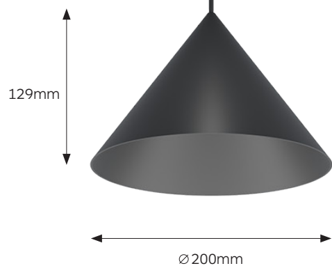
DELTA 200 Watt: 14W Lumen: 1789lm
