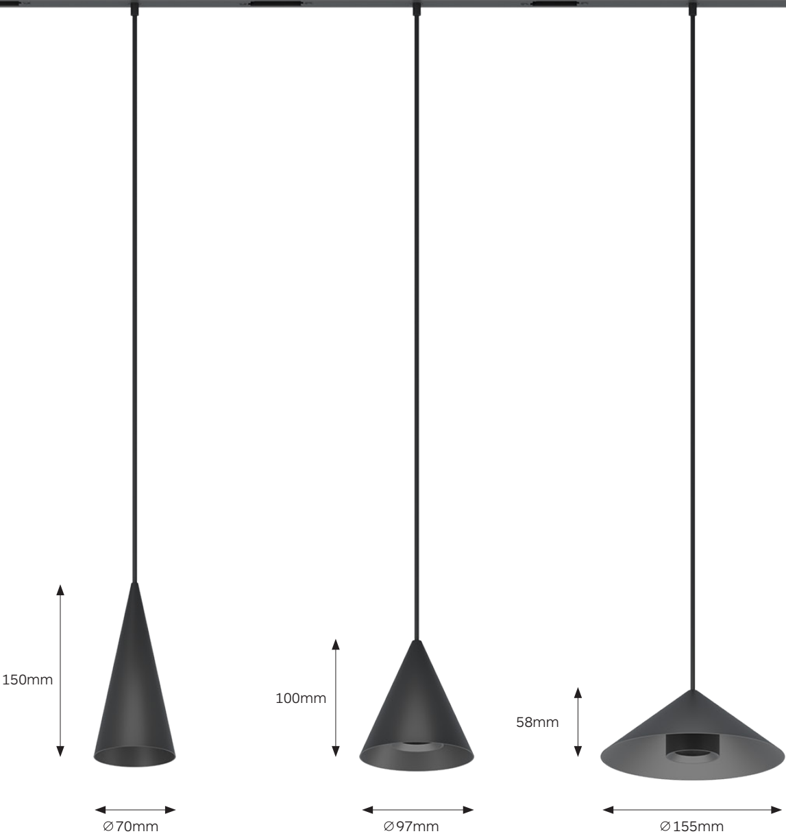
DELTA 70 Watt: 15.4W Beam Angle: 13°-44°
