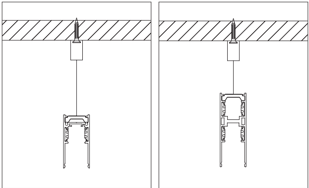
Pendant Up-Down Pendant
